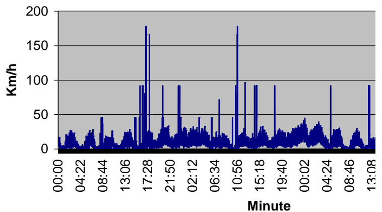
Vitesse du vent [Km/h] par minute pour Juil
